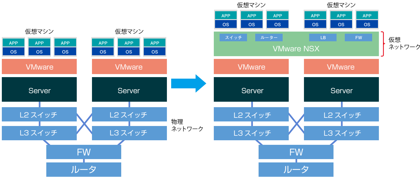
仮想マシンに合わせて、物理ネットワークの変更が必要
